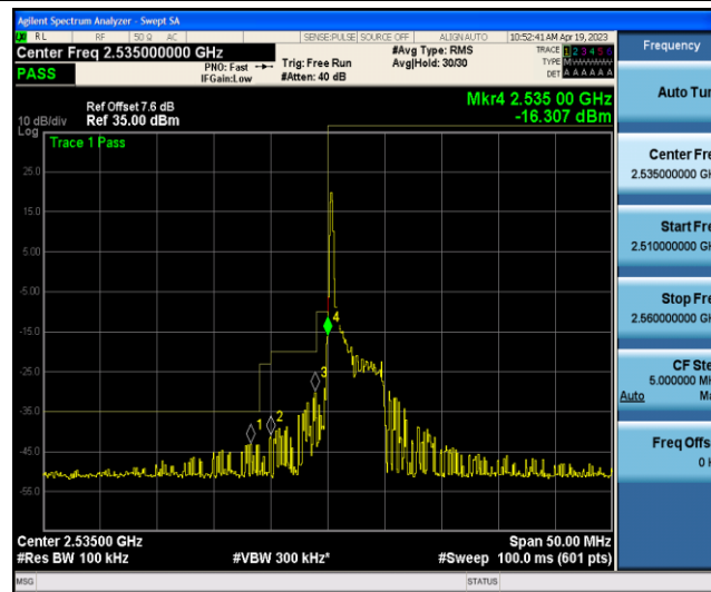
Band41-5MHz-QPSK-40065-1RB#24
