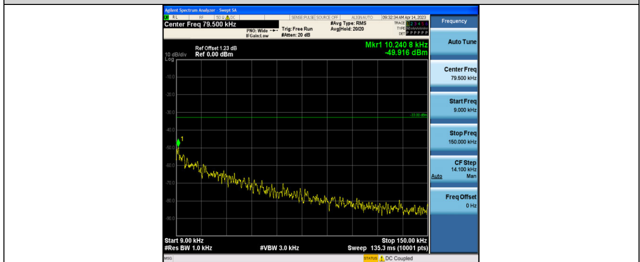
GSM850-190-0.009~0.15MHz
