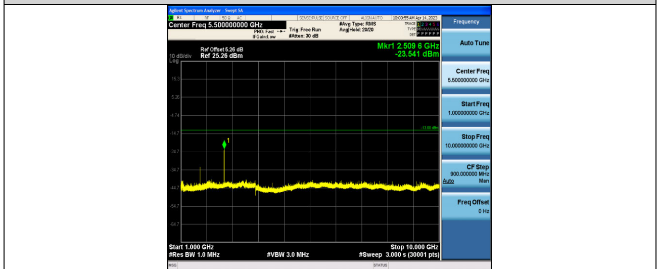
GPRS850-190-1000~10000MHz
