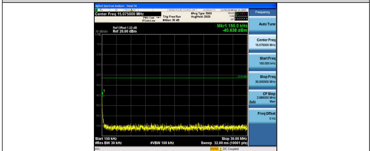
EGPRS1900-810-0.15~30MHz
