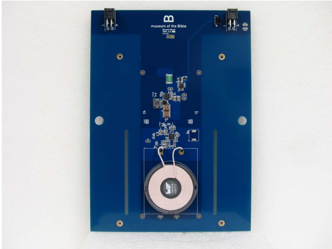
Dock Module Top
