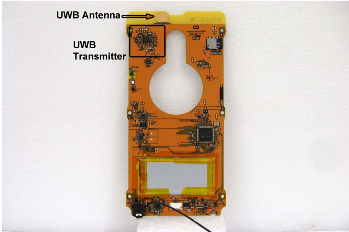
Docent Module Front Side
