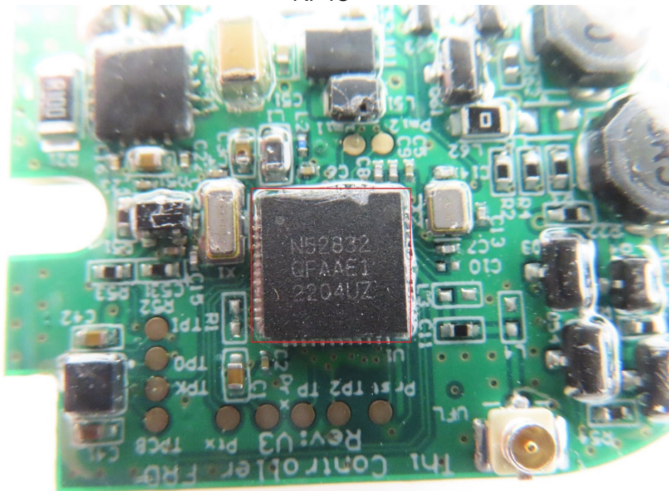
RF IC
