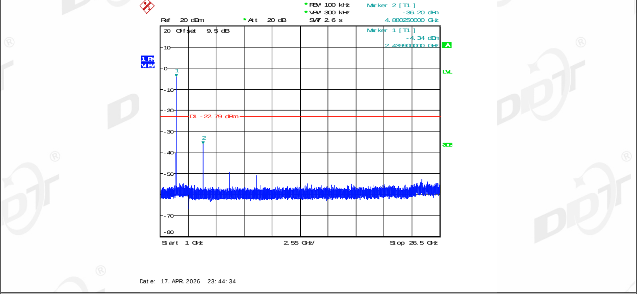
BLE 1M Ant2 2440 0-Reference
