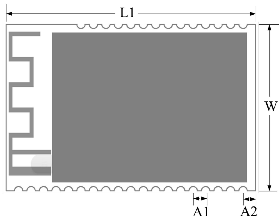
Fig. 9-1 Physical Dimensions of SZU06A2
