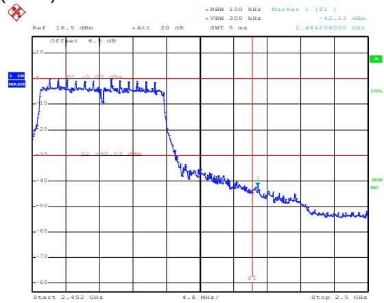
802.11n(HT20)
