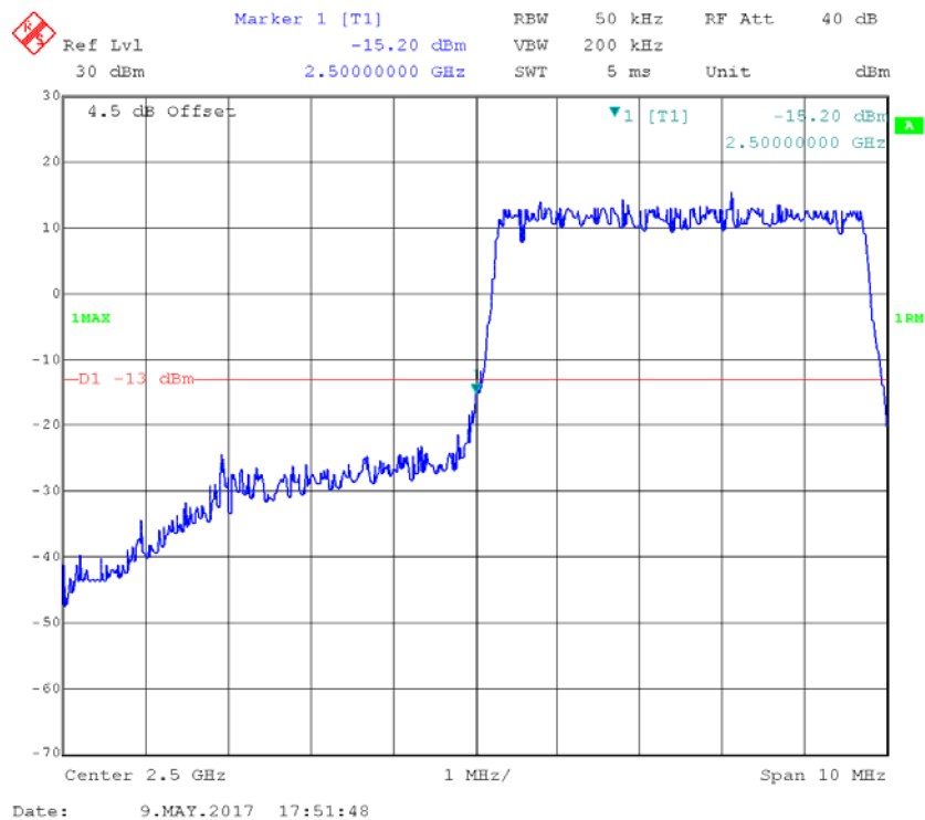
QPSK_5MHz_25 RB_Right
