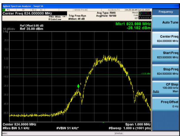
GSM 850-LCH-EPRS
