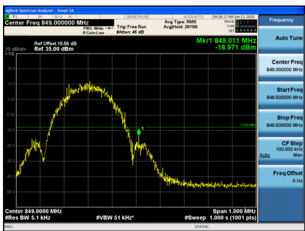
GSM 850-HCH-EGPRS
