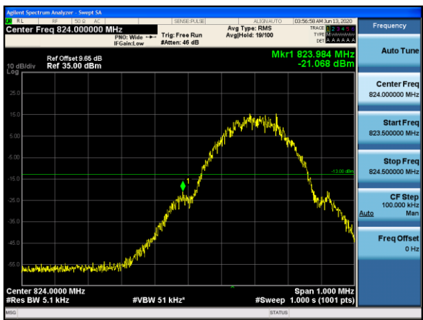
GSM 850-LCH-GSM
