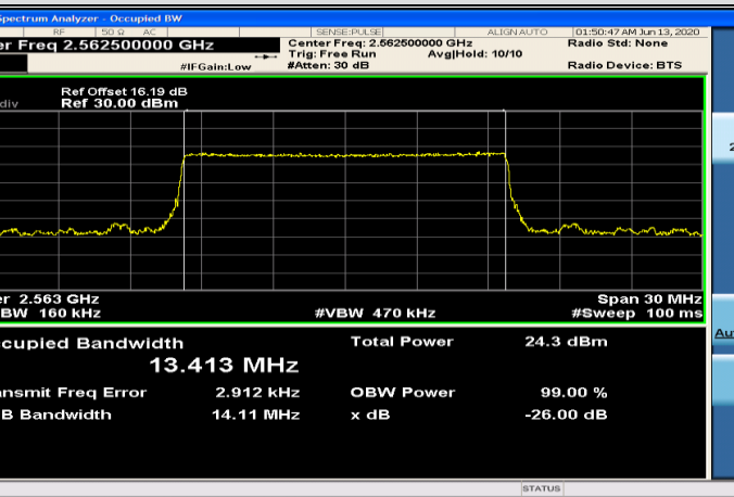
HCH_QPSK_75RB#0
