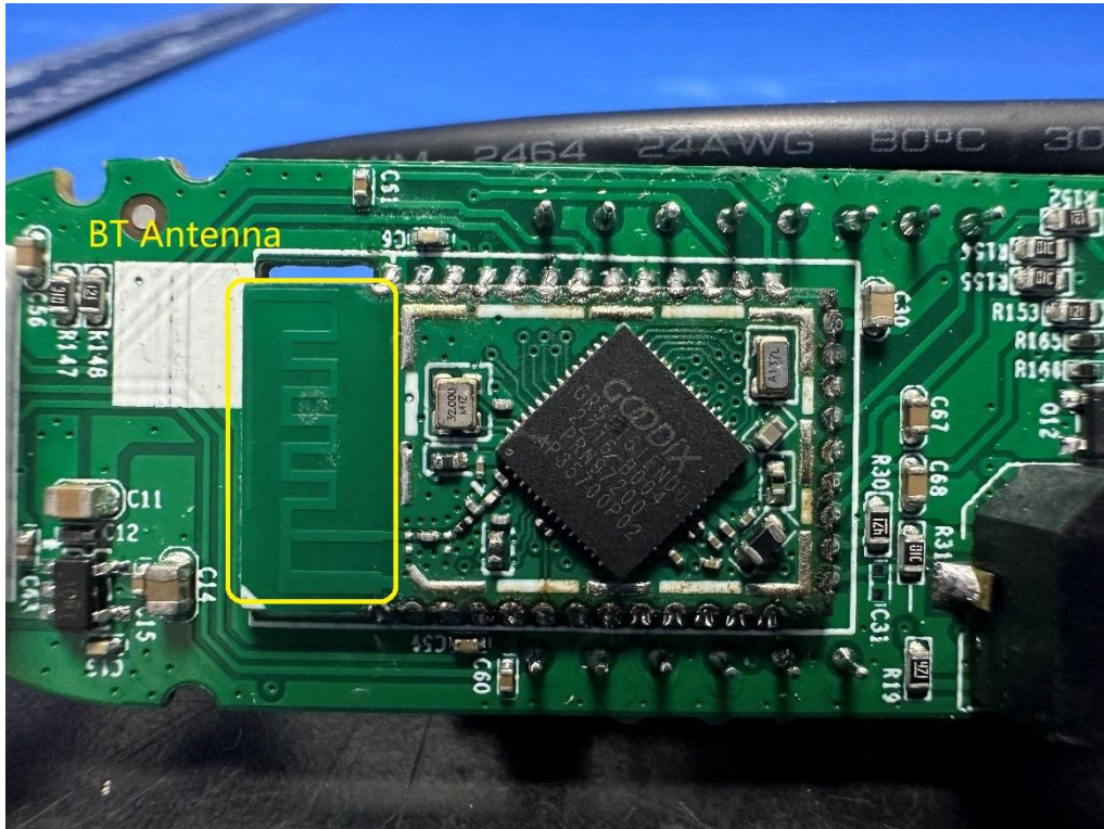
(5) EUT Photo
