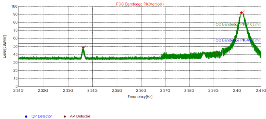
BLE_1M_2402_Ant1/ Vertical
