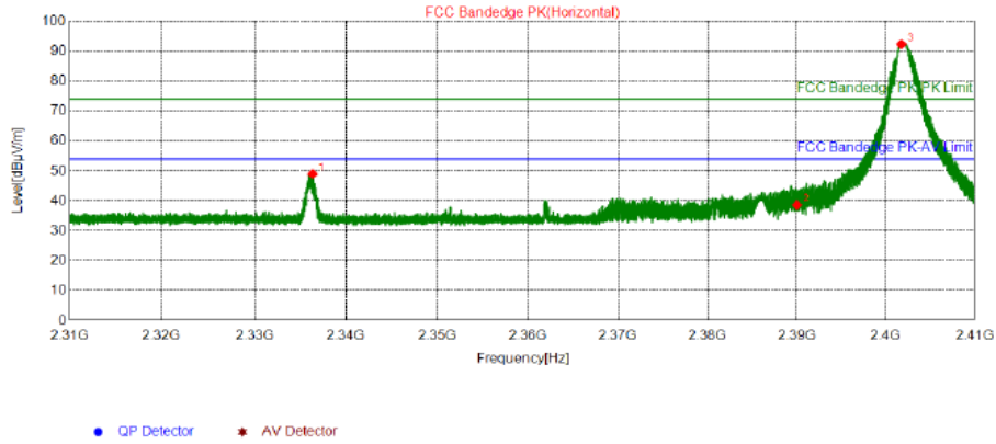
BLE_1M_2402_Ant1/ Horizontal
