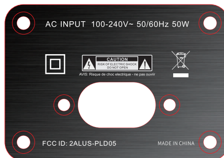
AU-4电源面板
