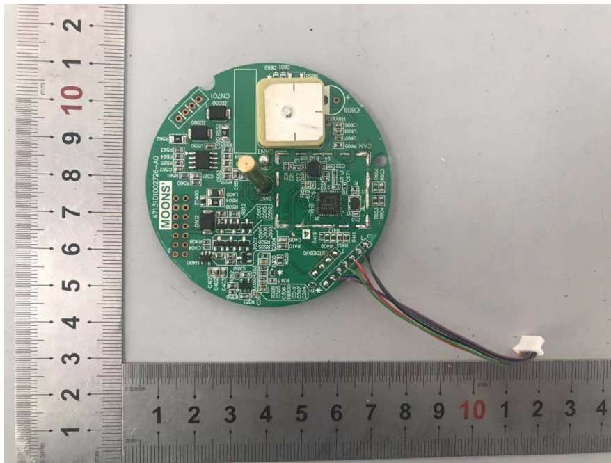
EUT - PCB-1 Top Chip View-1
