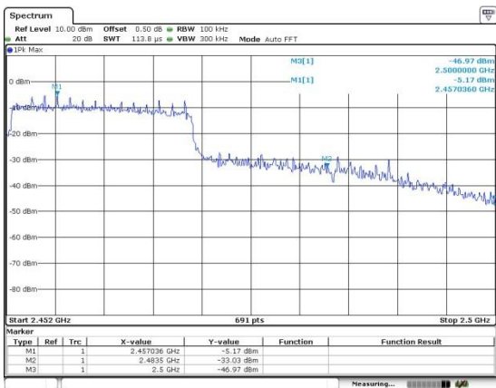
CH09-Bandedge
