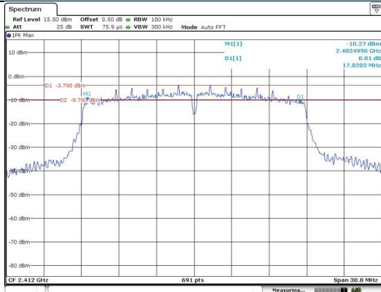
CH01
