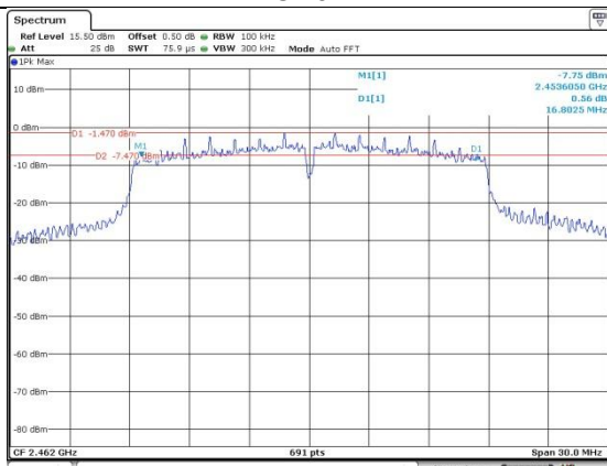
CH11
