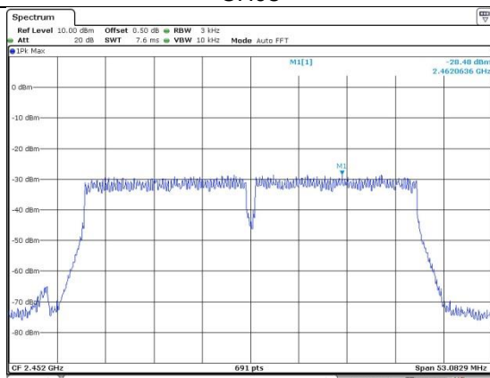
CH09
