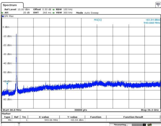
CH09-SE
