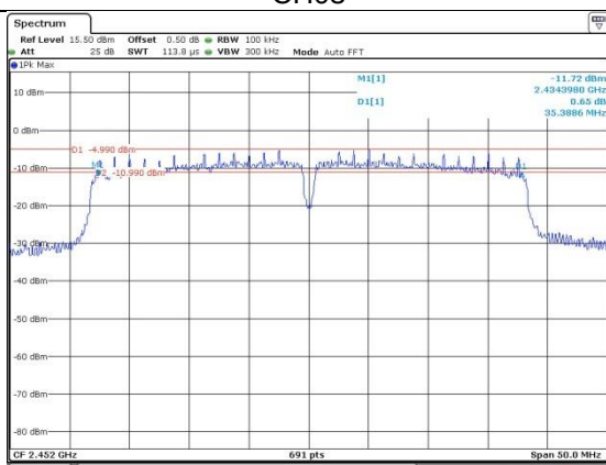
CH09
