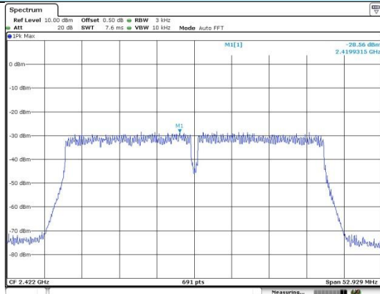
CH03
