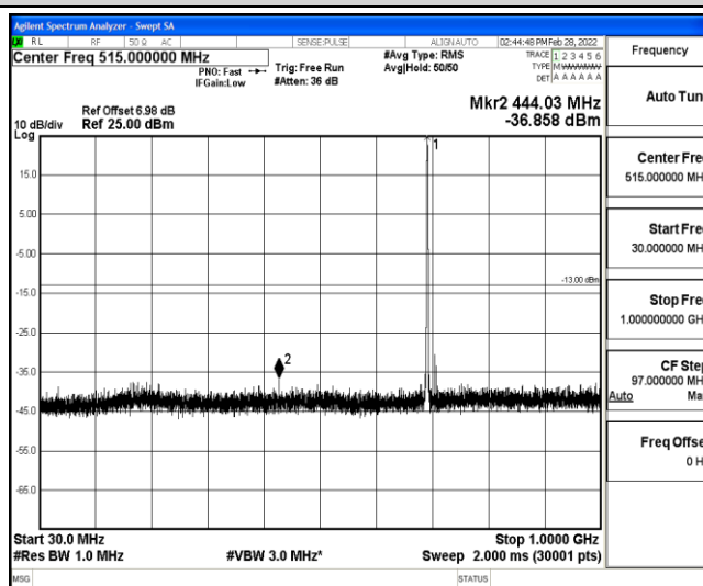
Band12-1.4MHz-16QAM-23017-1-0-Low-30-1000--36.86-PASS
