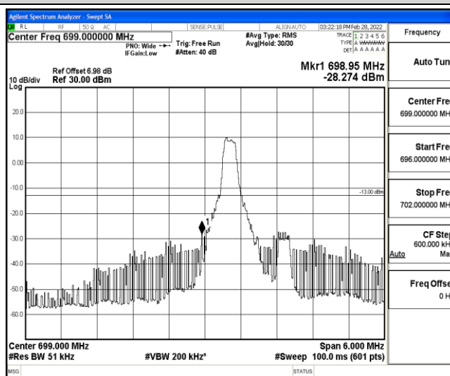
Band12-3MHz-QPSK-23025-1-0-Low--28.27-PASS
