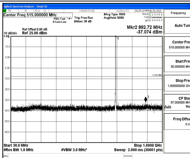
Band12-3MHz-QPSK-23025-1-0-Low-30-1000--37.07-PASS
