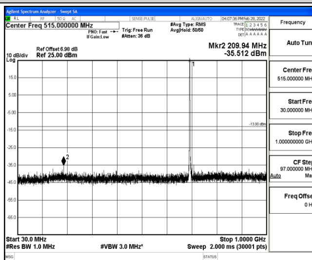
Band12-5MHz-QPSK-23035-1-0-Low-30-1000--35.51-PASS
