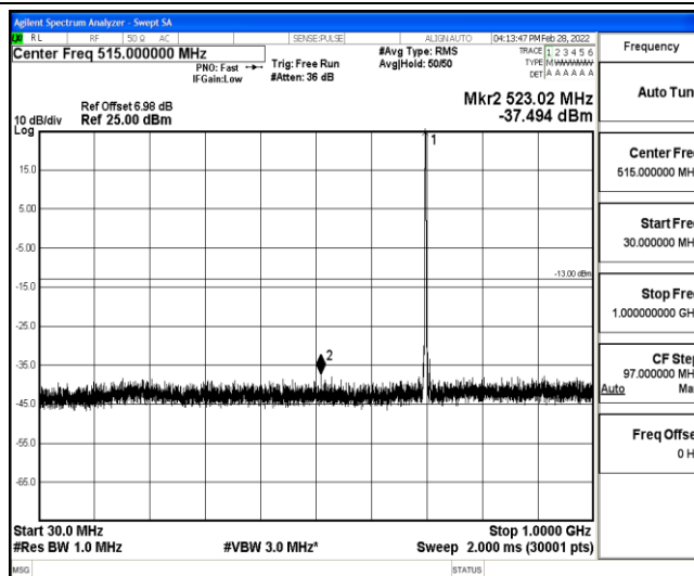
Band12-5MHz-16QAM-23095-1-0-Low-30-1000--37.49-PASS
