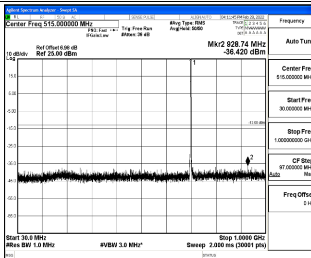
Band12-5MHz-QPSK-23095-1-0-Low-30-1000--36.42-PASS
