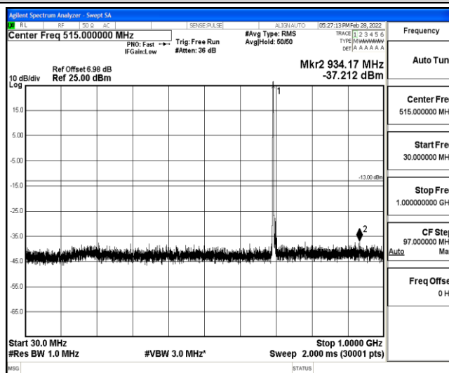
Band12-10MHz-QPSK-23060-1-0-Low-30-1000--37.21-PASS
