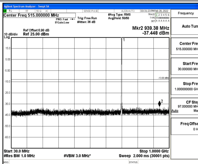
Band12-3MHz-16QAM-23095-1-0-Low-30-1000--37.45-PASS
