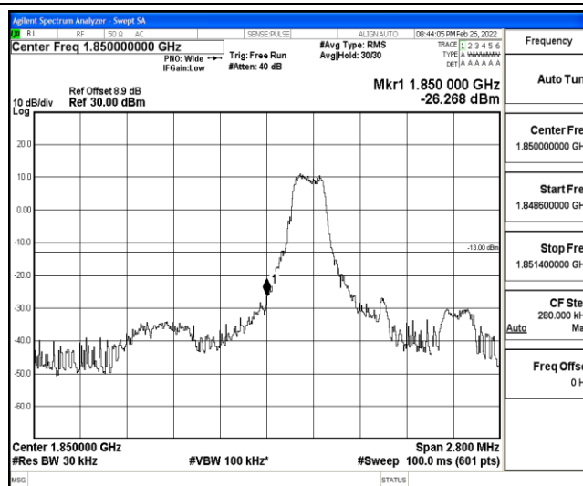
Band25-1.4MHz-QPSK-26047-1-0-Low--26.27-PASS
