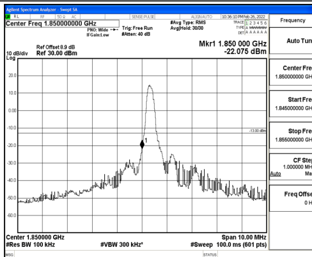
Band25-5MHz-QPSK-26065-1-0-Low--22.07-PASS
