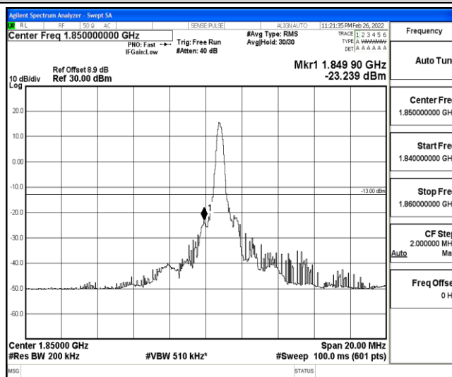
Band25-10MHz-16QAM-26090-1-0-Low--23.24-PASS
