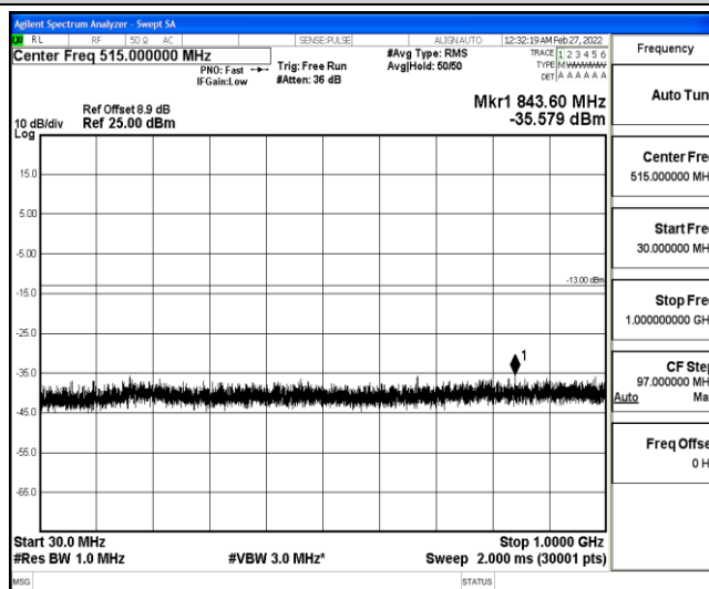
Band25-20MHz-QPSK-26140-1-0-Low-30-1000--35.58-PASS
