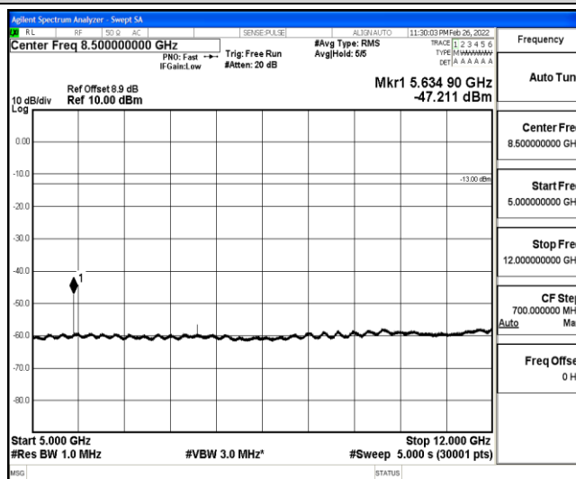
Band25-10MHz-QPSK-26365-1-0-Low-5000-12000--47.21-PASS
