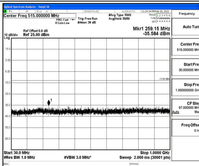
Band25-10MHz-QPSK-26090-1-0-Low-30-1000--35.58-PASS
