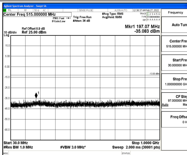
Band25-20MHz-16QAM-26365-1-0-Low-30-1000--35.08-PASS
