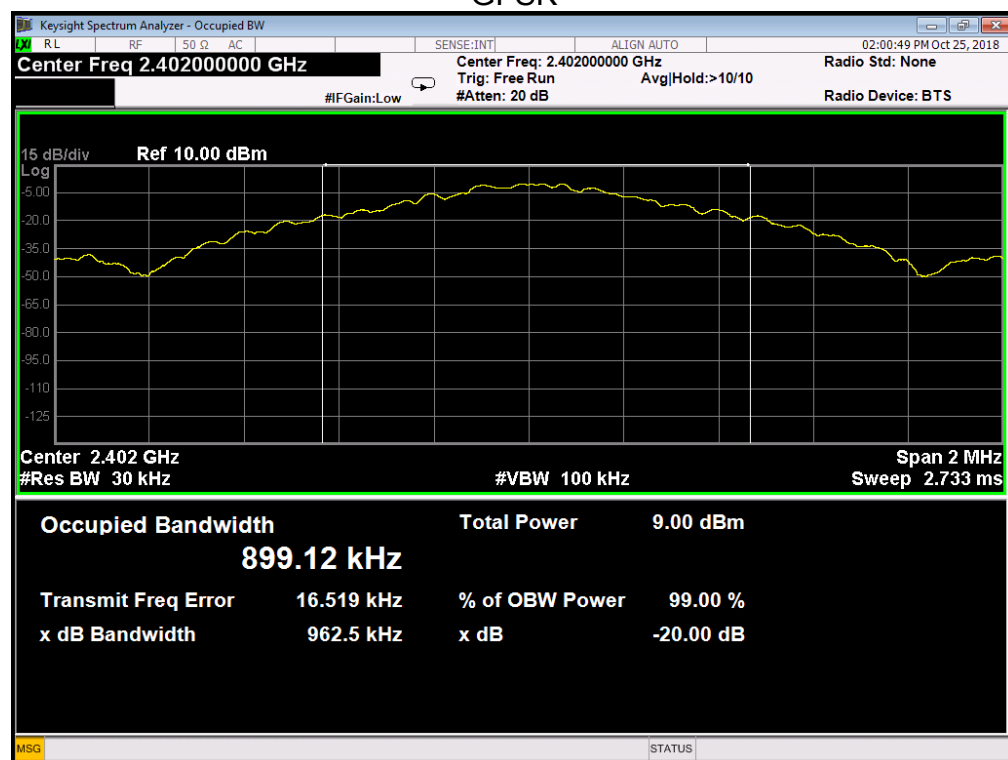
GFSK
