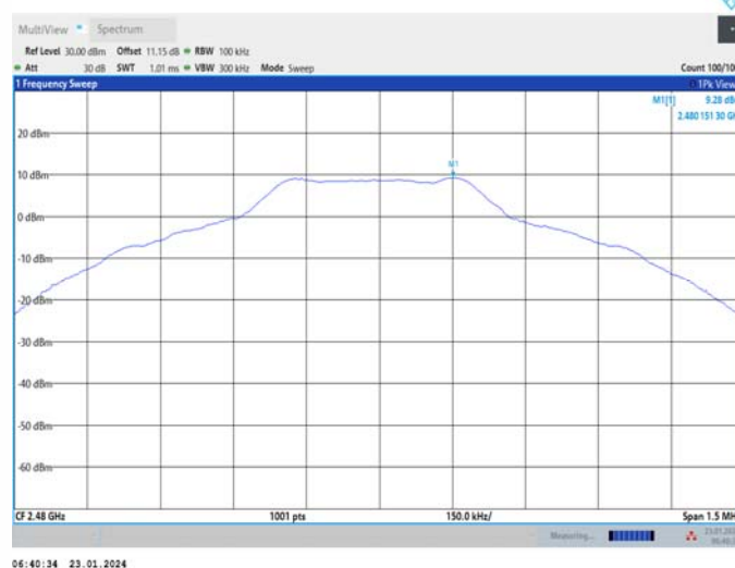
DH5_Ant1_2480
