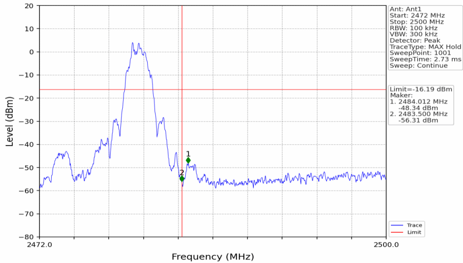
2M_HCH_2480MHz_Ant1_NTNV
