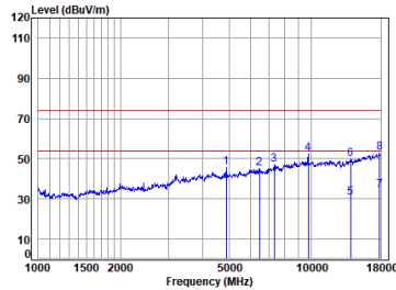
Right BT_DH5_TX_CH_39_Horizontal
