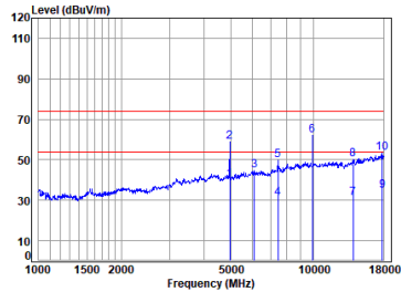
Left BT_DH5_TX_CH_78_Horizontal
