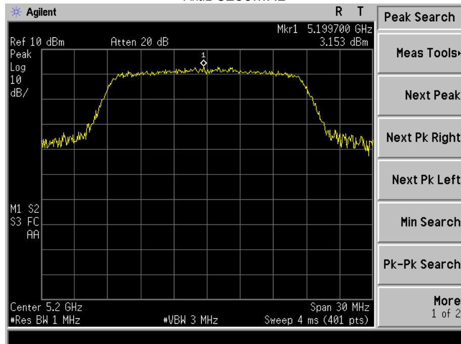
Ant.1 5200MHz
