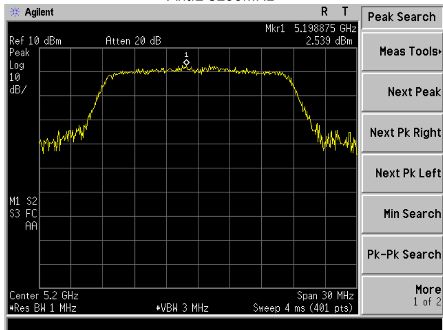
Ant.2 5200MHz
