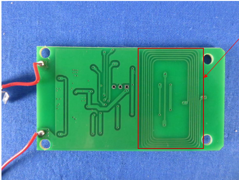
8MHz Antenna
