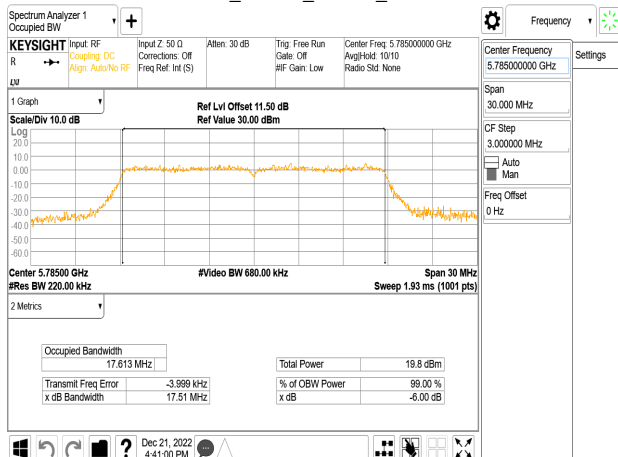
802.11n_20MHz_Chain0_5785MHz
