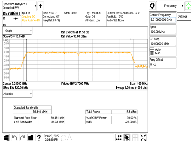
802.11ac_80MHz_Chain0_5210MHz
