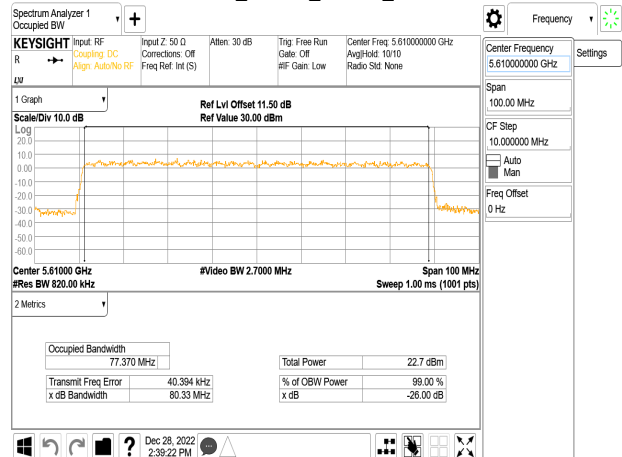
802.11ax_80MHz_Chain0_5610MHz
