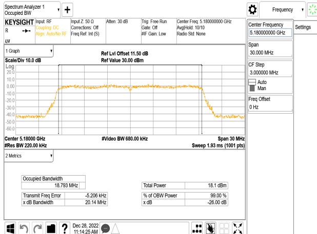
802.11ax_20MHz_Chain0_5180MHz
