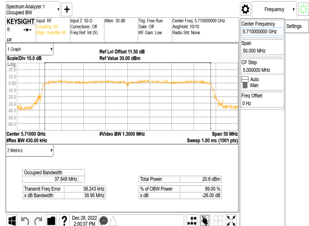
802.11ax_40MHz_Chain0_5710MHz
