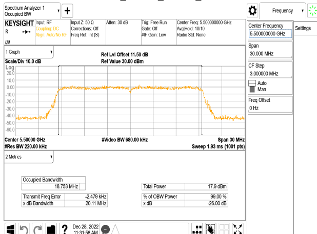
802.11ax_20MHz_Chain0_5500MHz
