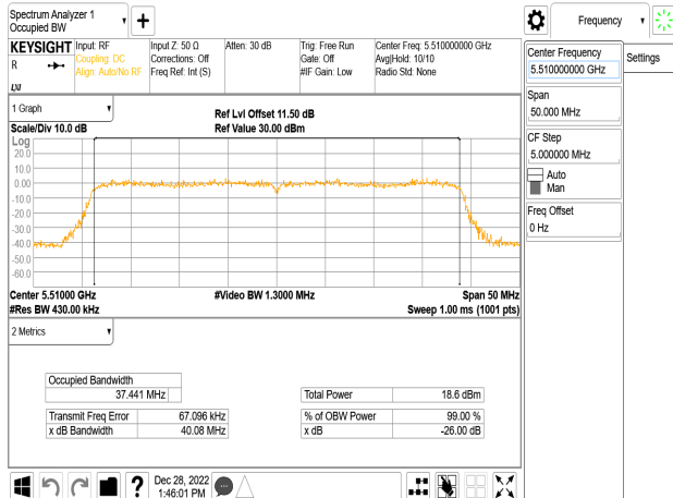
802.11ax_40MHz_Chain0_5510MHz
