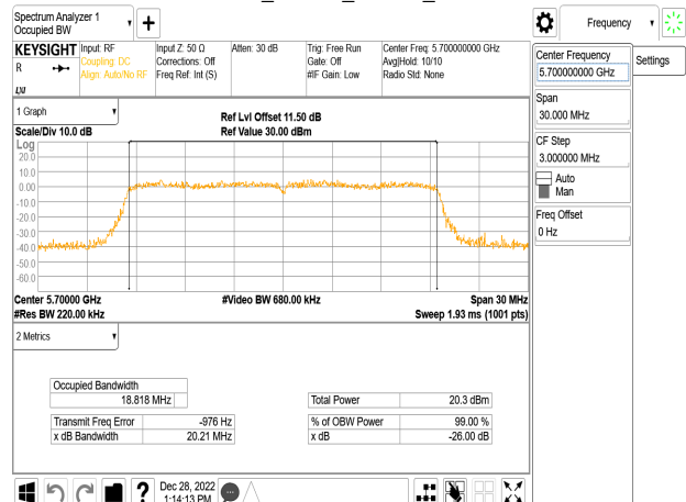
802.11ax_20MHz_Chain0_5700MHz
