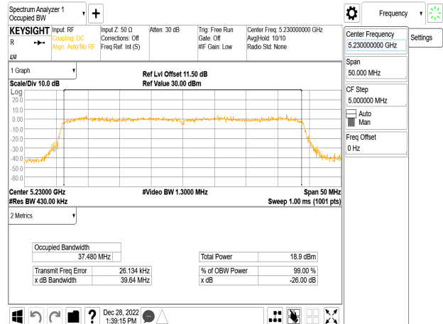
802.11ax_40MHz_Chain0_5230MHz
