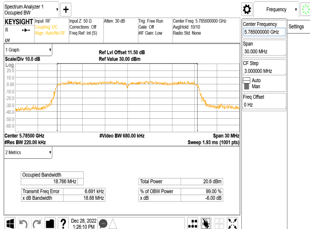
802.11ax_20MHz_Chain0_5785MHz
