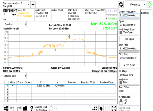
802.11ax_20MHz_Chain0_5220MHz_RU26_0
