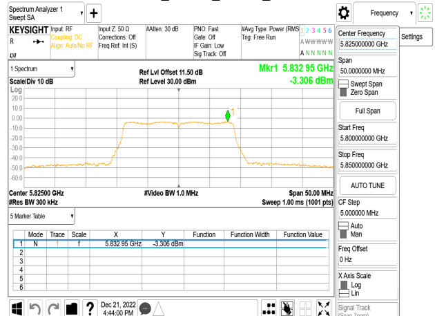
802.11n_20MHz_Chain0_5825MHz
