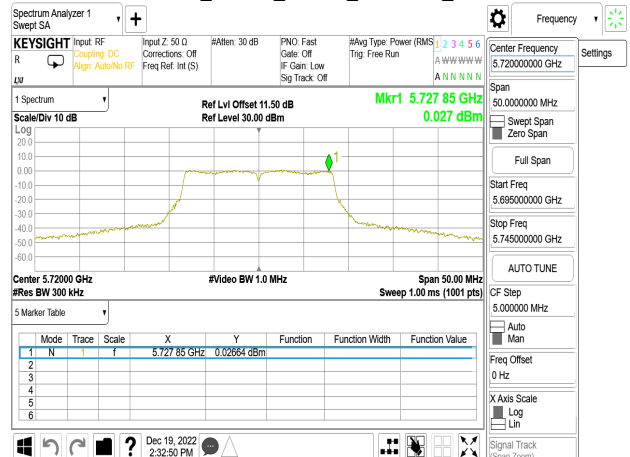
802.11a_20MHz_Chain0_5720MHz_UNII 3
