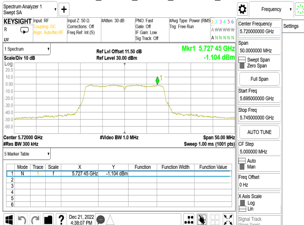
802.11n_20MHz_Chain0_5720MHz_UNII 3
