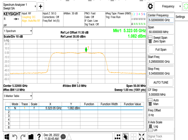
802.11ax_20MHz_Chain0_5320MHz_SU
