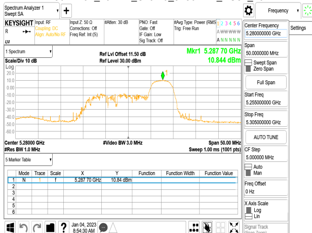
802.11ax_20MHz_Chain0_5280MHz_RU52_40
