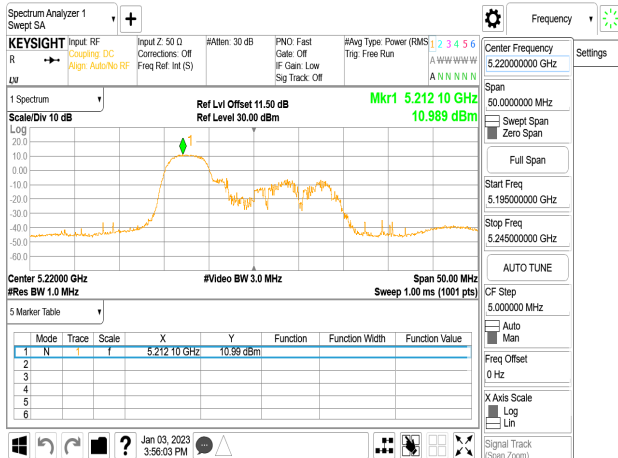
802.11ax_20MHz_Chain0_5220MHz_RU52_40
