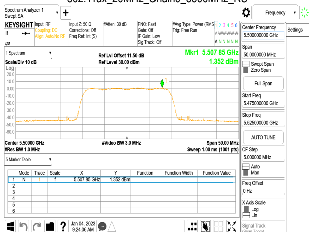
802.11ax_20MHz_Chain0_5500MHz_RU106_53
