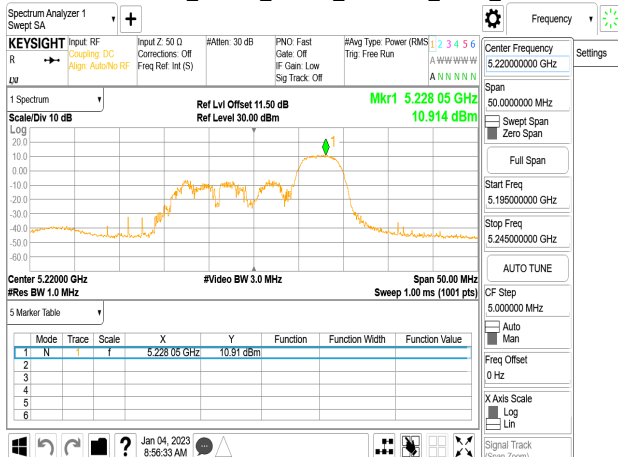
802.11ax_20MHz_Chain0_5220MHz_RU52_40
