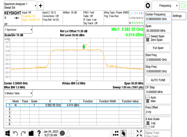
802.11ax_20MHz_Chain0_5580MHz_SU
