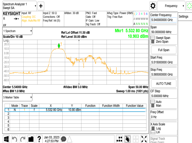
802.11ax_20MHz_Chain0_5540MHz_RU52_40
