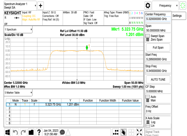
802.11ax_20MHz_Chain0_5320MHz_RU106_53
