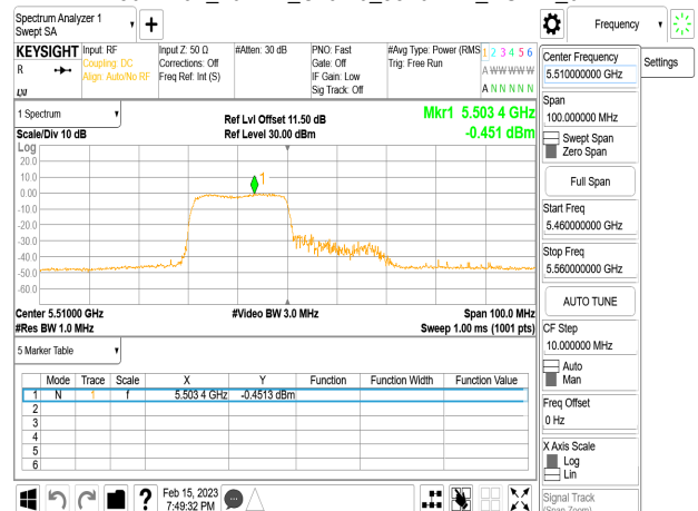
802.11ax_40MHz_Chain0_5510MHz_RU242_62
