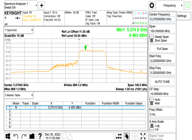
802.11ax_40MHz_Chain0_5270MHz_SU
