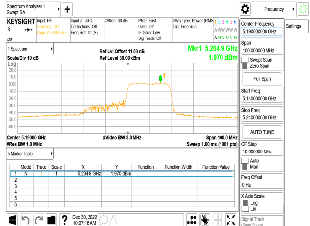
802.11ax_40MHz_Chain0_5190MHz_SU
