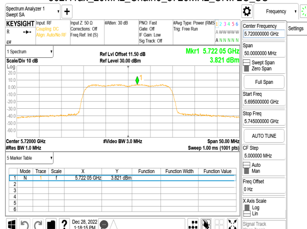
802.11ax_20MHz_Chain0_5720MHz_UNII 2C_SU
