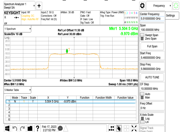
802.11ax_40MHz_Chain0_5510MHz_RU242_61
