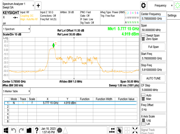
802.11ax_20MHz_Chain0_5785MHz_RU26_8
