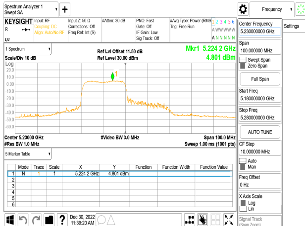
802.11ax_40MHz_Chain0_5230MHz_RU242_62
