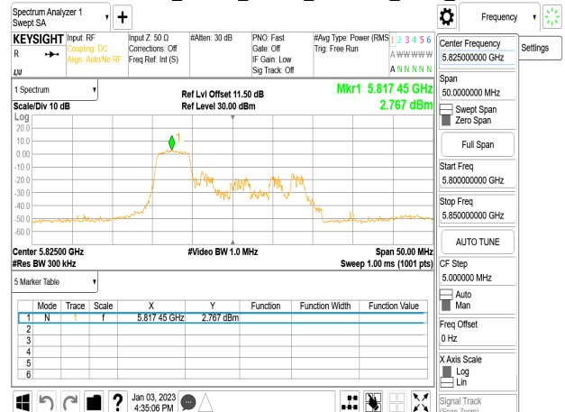
802.11ax_20MHz_Chain0_5825MHz_RU52_37
