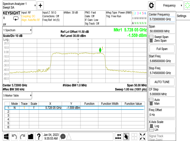
802.11ax_20MHz_Chain0_5720MHz_UNII 3 SU
