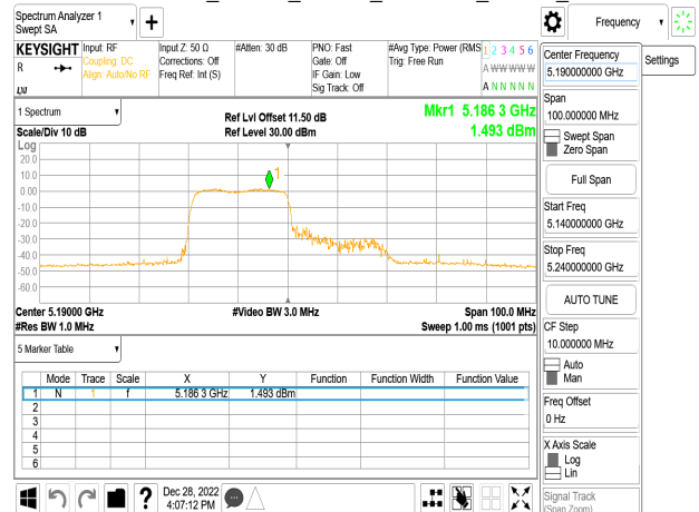
802.11ax_40MHz_Chain0_5190MHz_RU242_62
