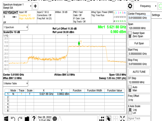
802.11ax_80MHz_Chain0_5610MHz_RU484_66
