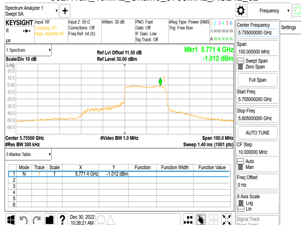
802.11ax_40MHz_Chain0_5755MHz_SU
