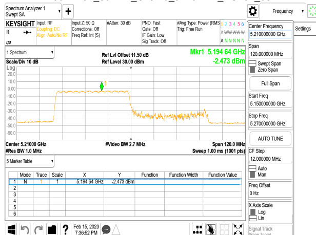
802.11ax_80MHz_Chain0_5210MHz_RU484_66
