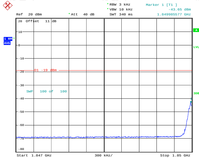
Band2 GSM UL Left Side Pre AGC
