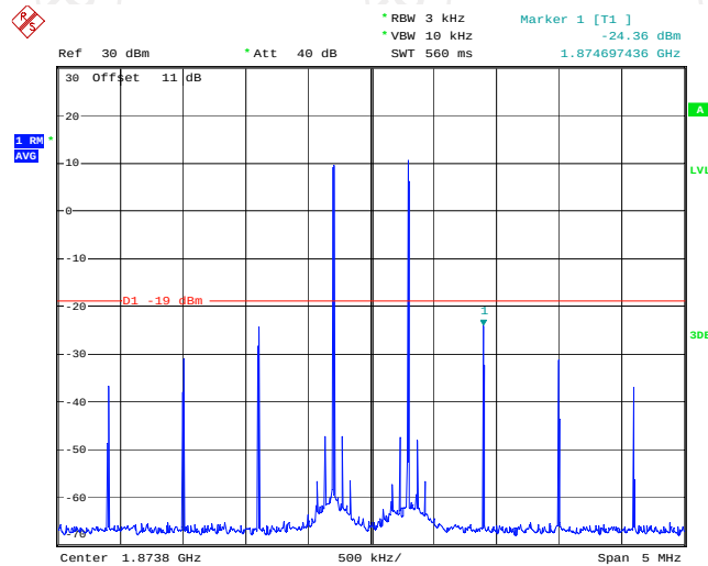
Band2 Pre AGC, UL
