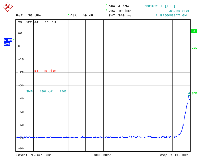
Band2 GSM UL Left Side Max. Input
