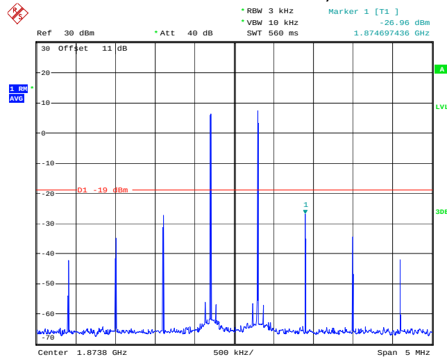
Band2 AGC +10dB, UL
