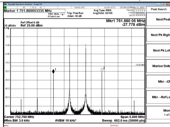
Upper 700MHz band AGC+10dB, DL
