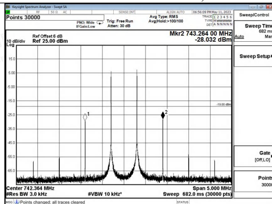
Lower 700MHz band AGC+10dB, DL
