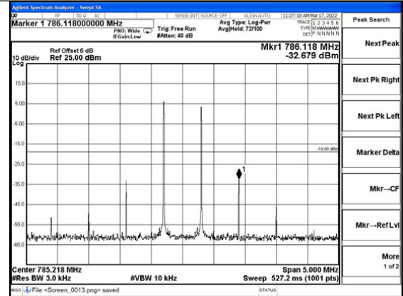
Upper 700MHz band AGC+10dB, UL
