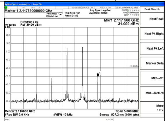
AWS Band AGC+10dB, DL
