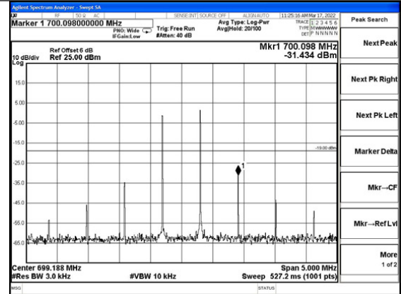
Lower 700MHz band AGC+10dB, UL
