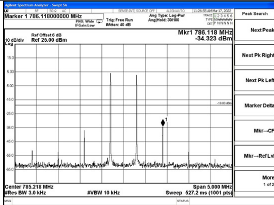
Upper 700MHz band Pre AGC, UL
