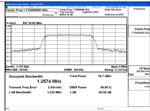
CDMA-AWS band UL output
