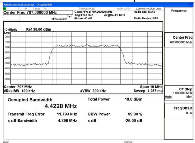
Lower 700MHz UL output
