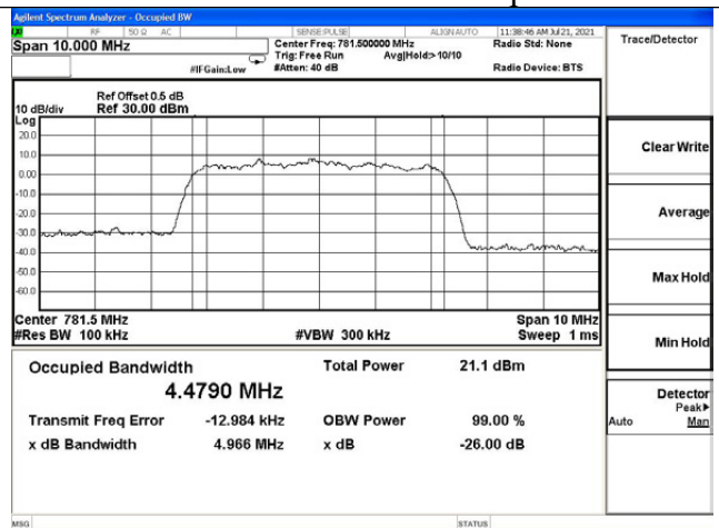
Upper 700MHz UL output
