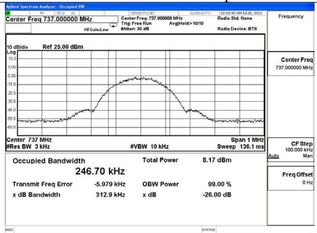
Lower 700MHz DL output
