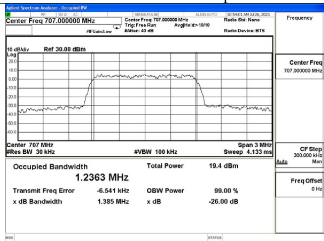
Lower 700MHz UL output
