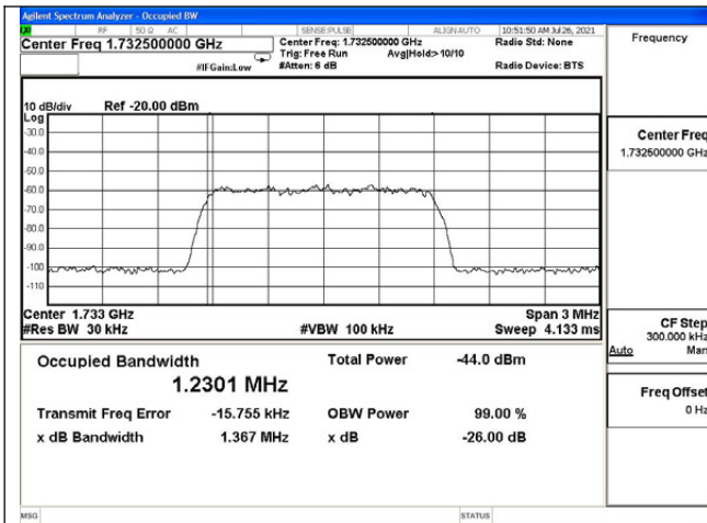
AWS band UL input
