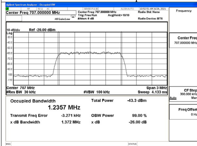
Lower 700MHz band UL input
