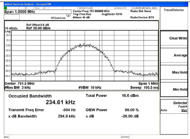
Upper 700MHz DL output
