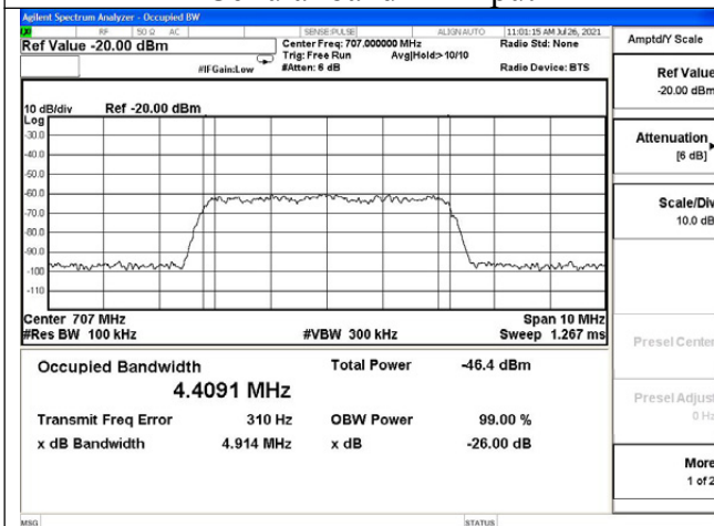
Lower 700MHz band UL input
