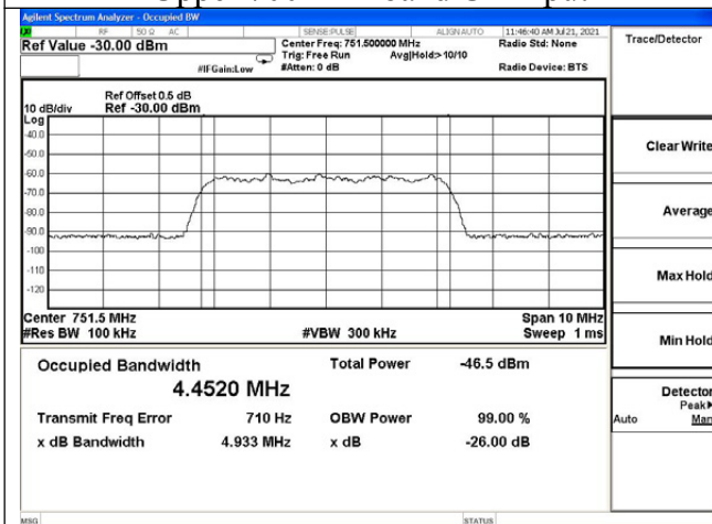
Upper 700MHz band DL input
