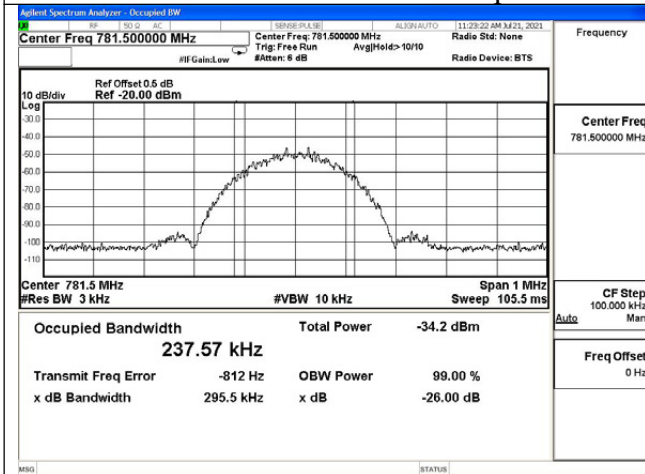
Upper 700MHz band UL input
