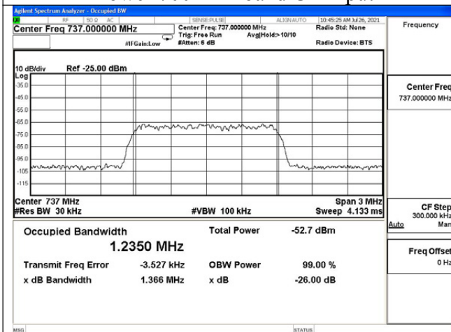
Lower 700MHz band DL input
