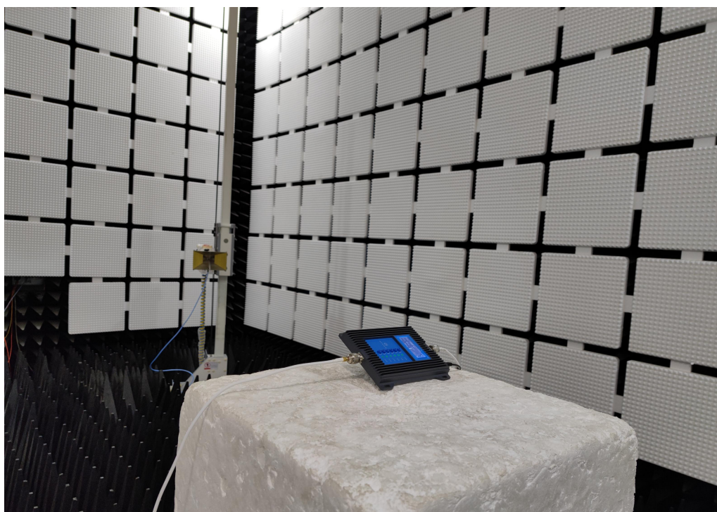
Fig. 5 (Above 1GHz)
