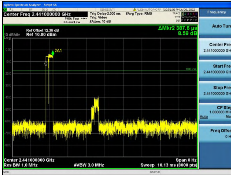
2DH3_Ant1_Hop
