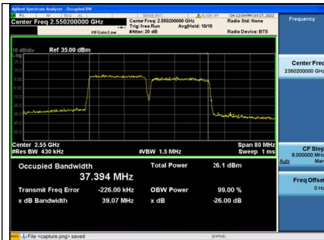
Band7C / 20MHz+20MHz / QPSK/ High CH
