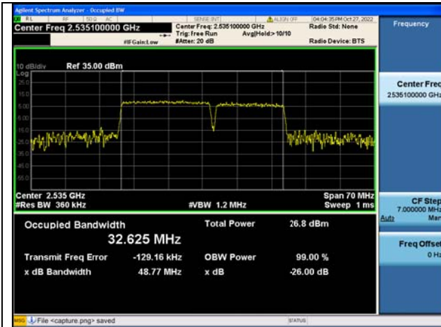
Band7C / 20MHz+15MHz / QPSK/ Mid CH
