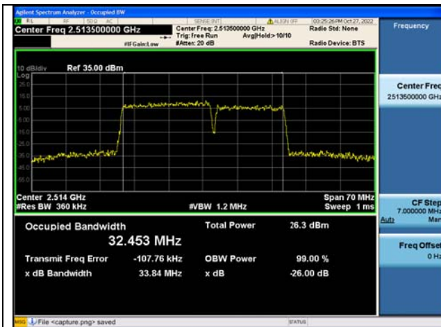
Band41C / 20MHz+15MHz / QPSK/ Low CH
