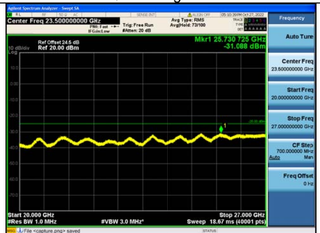
Band7C-20G-27G / 20MHz+10MHz /100RB+50RB/ QPSK / High CH
