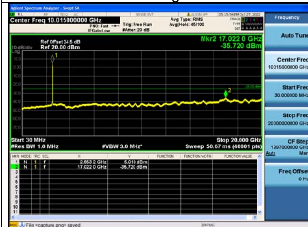
Band7C-30M-20G / 15MHz+10MHz /75RB+50RB/ QPSK / High CH
