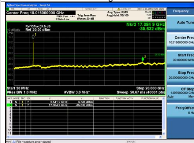
Band7C-30M-20G / 15MHz+15MHz /75RB+75RB/ QPSK / High CH
