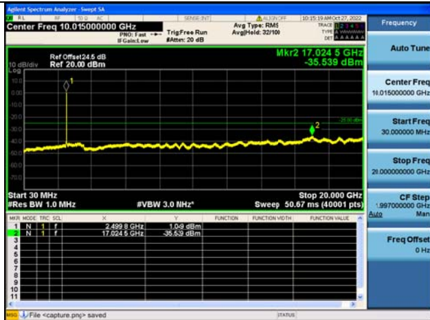
Band41C-30M-20G / 20MHz+10MHz /100RB+50RB/ QPSK / LOW CH
