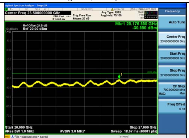
Band7C-20G-27G / 15MHz+20MHz / 75RB+100RB / QPSK / Mid CH
