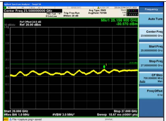
Band7C-20G-27G / 20MHz+15MHz / 100RB+75RB / QPSK / Mid CH
