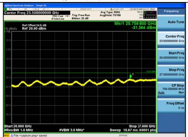
Band41C-20G-27G / 5MHz+20MHz /25RB+100RB/ QPSK / LOW CH
