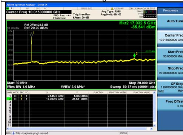
Band7C-30M-20G / 15MHz+20MHz /75RB+100RB/ QPSK / High CH
