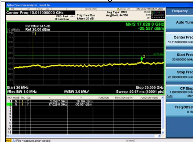
Band7C-30M-20G / 20MHz+10MHz / 1RB+1RB/ QPSK / High CH
