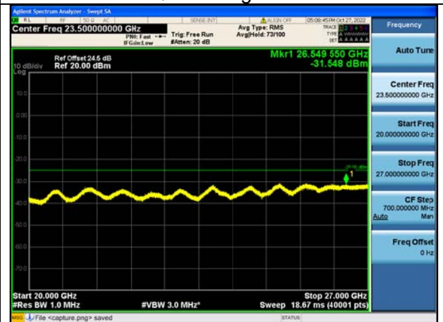
Band7C-20G-27G / 10MHz+20MHz / 50RB+100RB / QPSK / High CH
