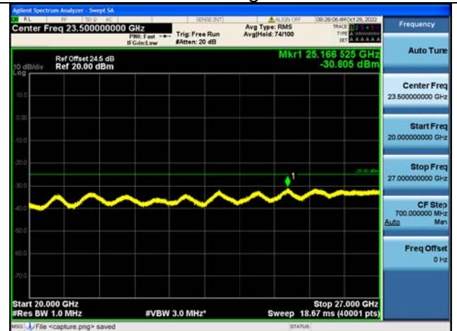
Band7C-20G-27G / 20MHz+15MHz / 1RB+1RB/ QPSK / High CH
