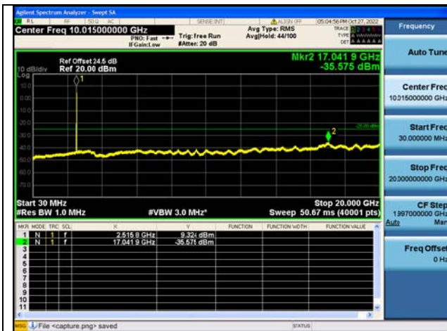
Band7C-30M-20G / 20MHz+20MHz / 1RB+1RB / QPSK / Mid CH
