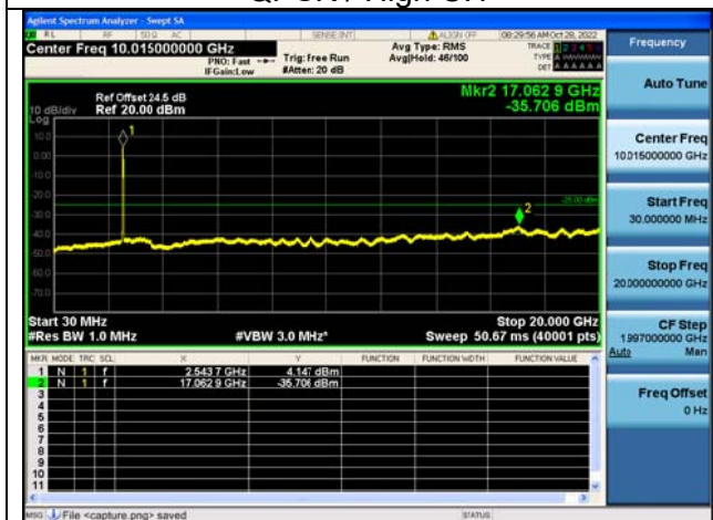
Band7C-30M-20G / 20MHz+20MHz /100RB+100RB/ QPSK / High CH
