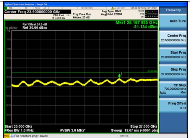
Band7C-20G-27G / 15MHz+10MHz / 1RB+1RB/ QPSK / High CH
