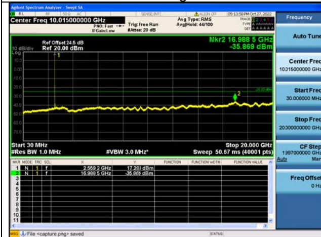
Band7C-30M-20G / 15MHz+10MHz / 1RB+1RB/ QPSK / High CH
