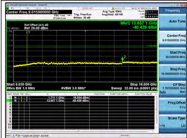
Band4 / 5MHz / Low CH / 64QAM
