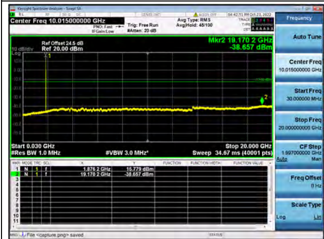
Band2 / 10MHz / Mid CH / 64QAM
