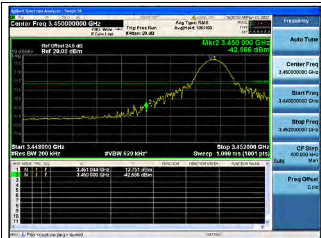
Band42 / 20MHz / Low CH / QPSK / 1 RB
