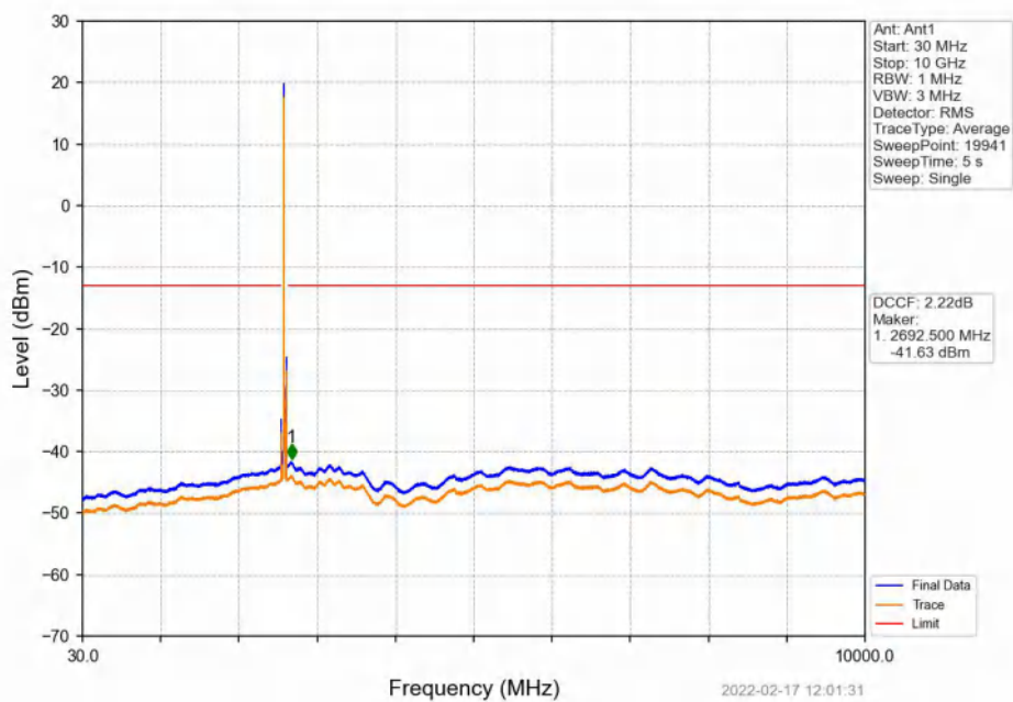
Band41_20MHz_QPSK_MCH_2605MHz_RB_1_0_NTNV
