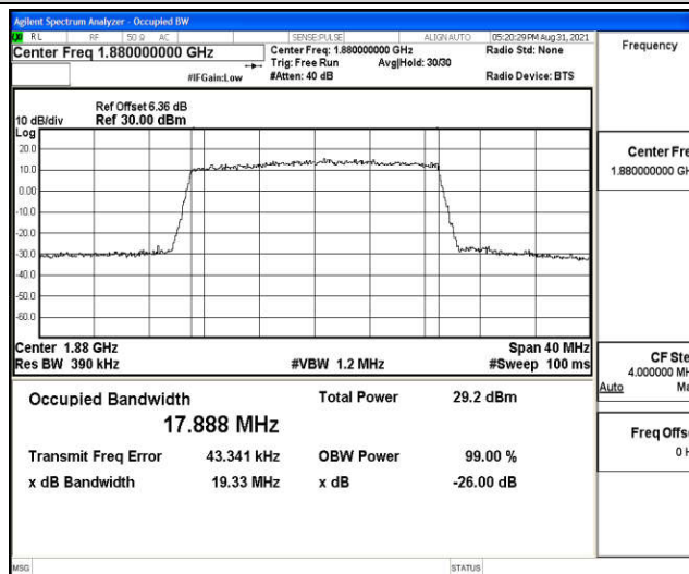
Band2-20MHz-16QAM-19100-100RB#0
