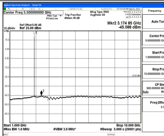
Band41-5MHz-QPSK-41565-1RB#0-Range5:10000~20000MHz
