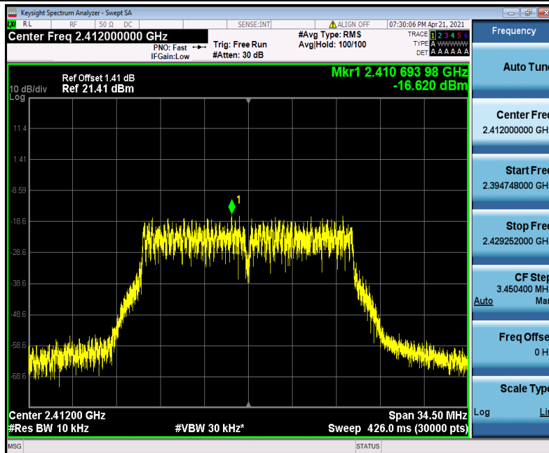
11G_Ant1_2412
