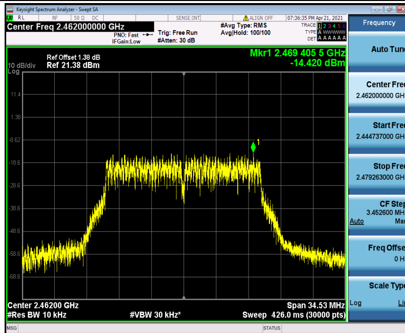
11G_Ant1_2462
