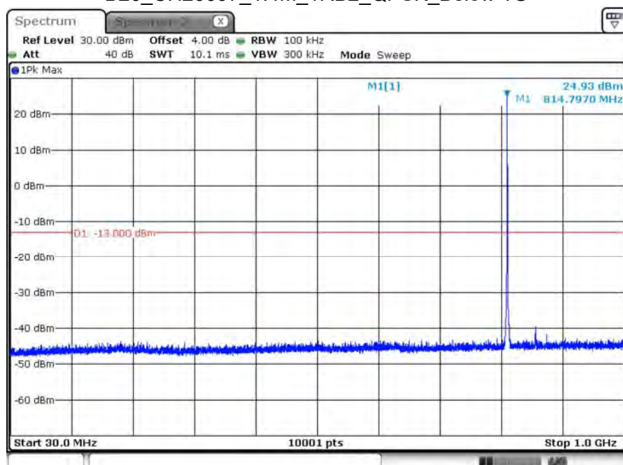
B26_CH26697_1.4M_1RB2_QPSK_Below 1G
