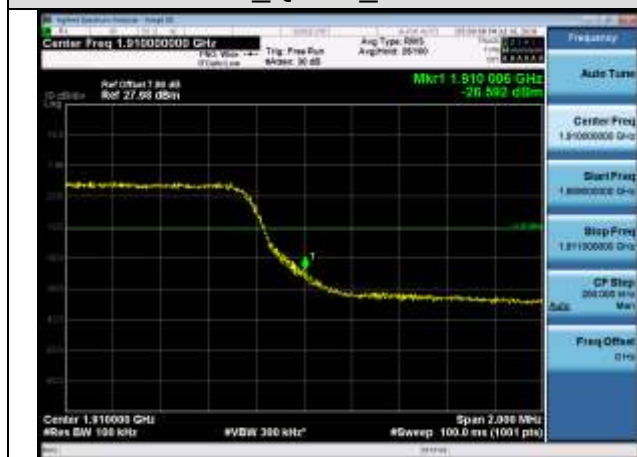
HCH_QPSK_25RB#0
